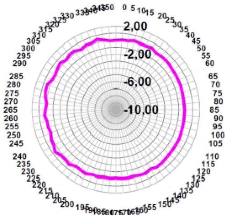
Freq. 900 MHz H-plane (dBi) V-pol
